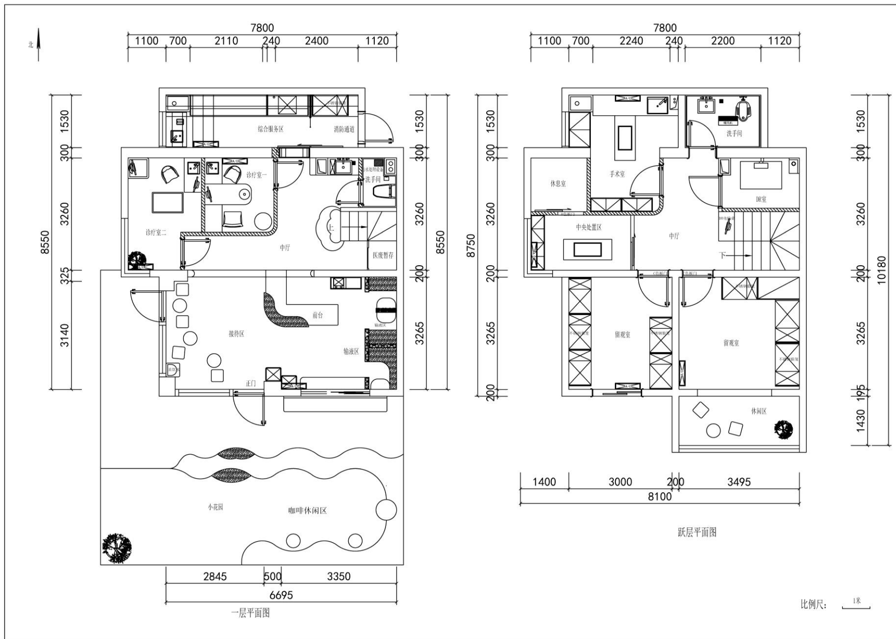
附图 3 建设项目平面布置图
