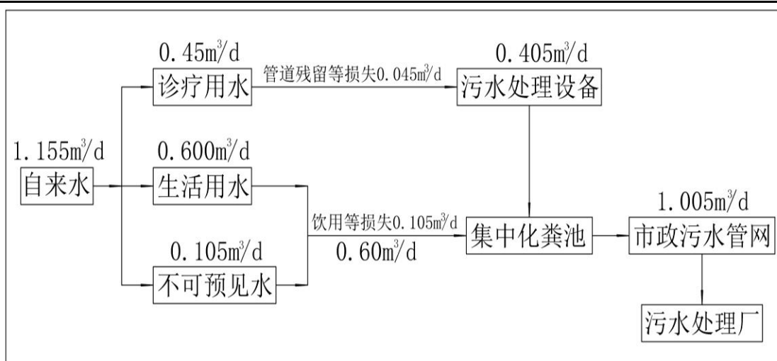
图 3 项目水平衡图
